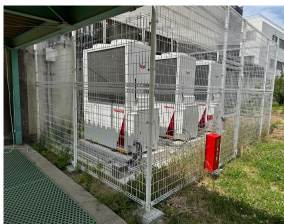
発電機能付き室外機設置状況
