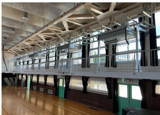
ギャラリー上の室内機設置状況 (前面に設置している機器が送風ファン)
