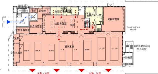
1階平面計画図
