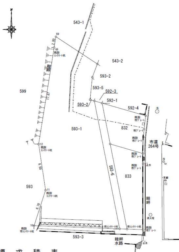
座 標 求 積 表
