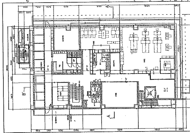
2階平面図
