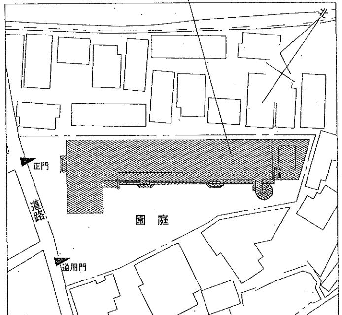
配置図 S=1:700
