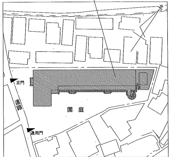
配置図 S=1:700
