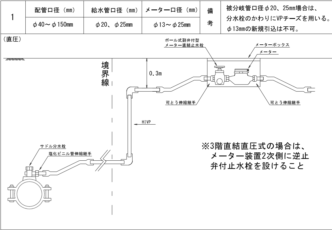
図-4.1.1 標準配管図 (メーター口径φ13～25 mm)
