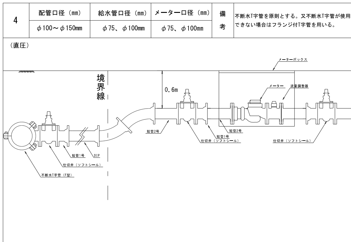
図-4.1.4 標準配管図 (メーター口径φ75～100 mm)
