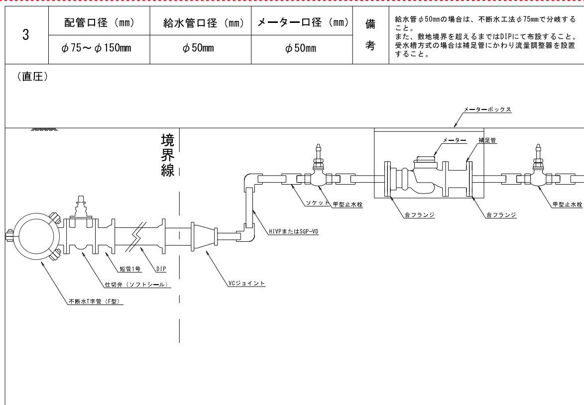
図-4.1.3 標準配管図 (メーター口径φ50 mm)
