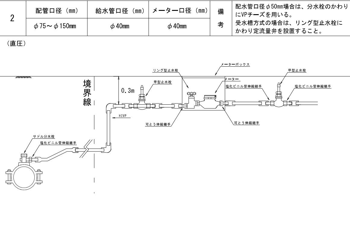
図-4.1.2 標準配管図 (メーター口径φ40 mm)
