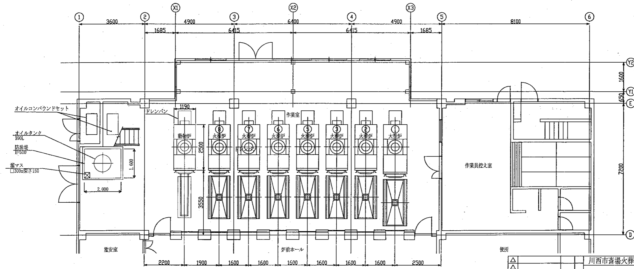
川西市斎場火葬炉更新工事完成平面図 (平成27年度)
