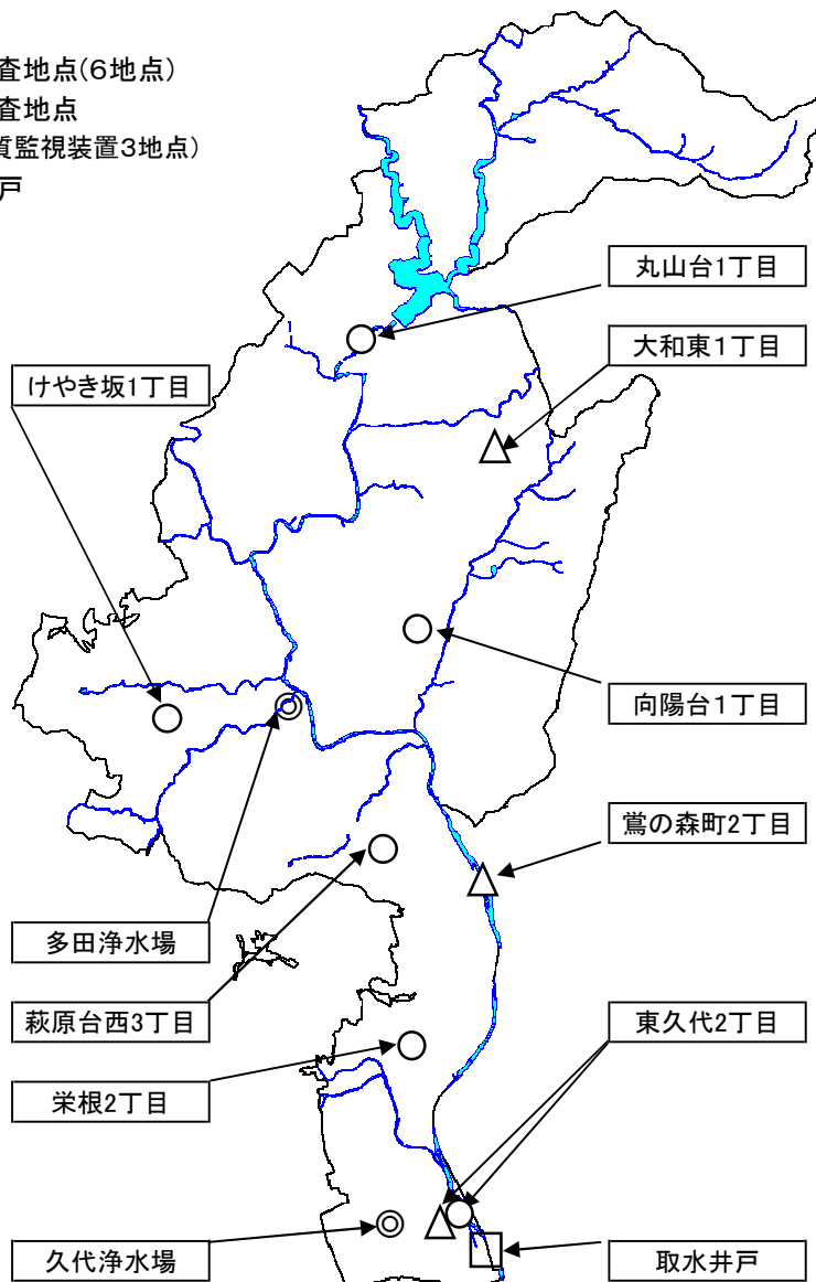
図-1 水道施設と水質検査地点
