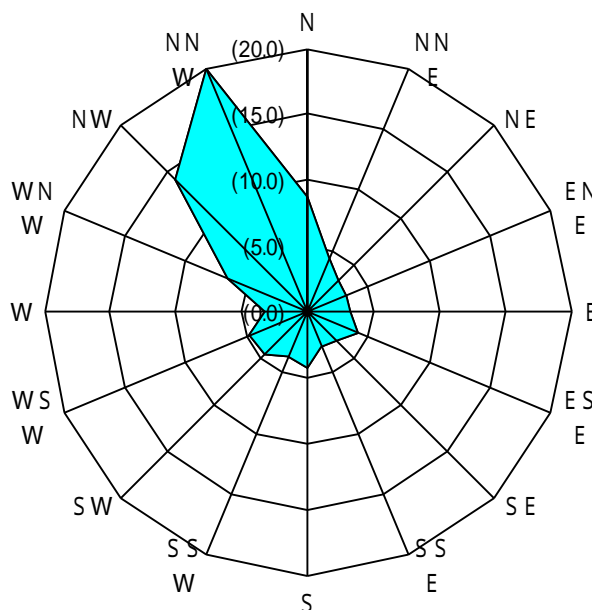
【図 5-14 令和2年度年間風配図（加茂自動車排気ガス測定局）】
