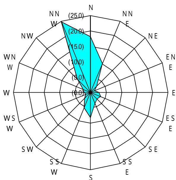
【図 5-7 令和2年度年間風配図(川西市役所局)】
