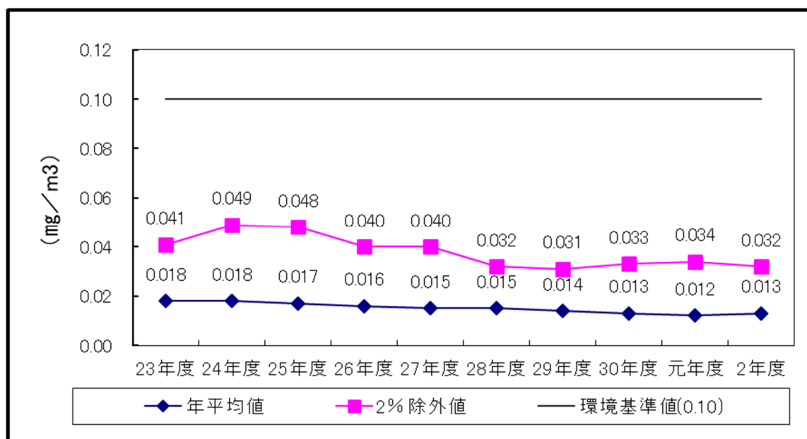
【図 5-3 川西市役所局浮遊粒子状物質濃度の経年変化 (年平均値及び日平均値の2%除外値)】
