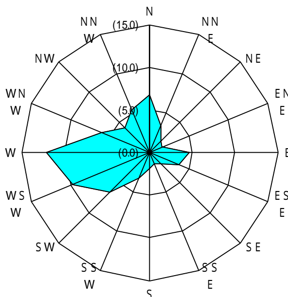
【図 5-15 令和2年度年間風配図 （川西文珠橋自動車排気ガス測定局）】
