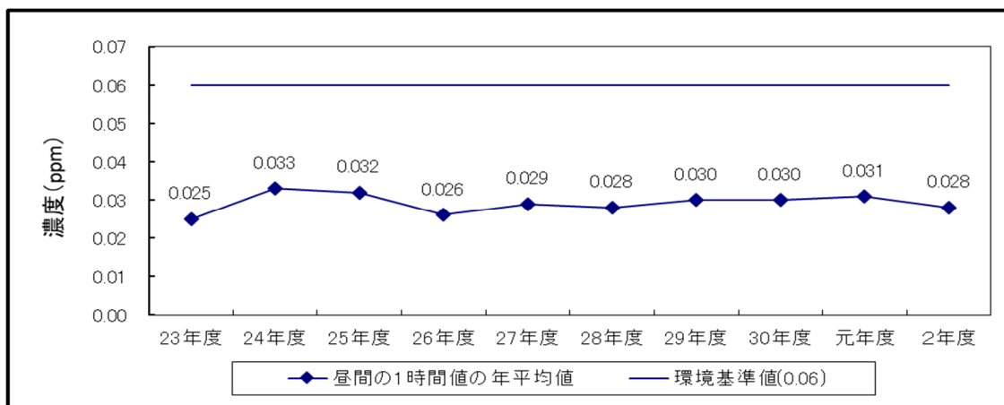
【図 5-5 川西市役所局光化学オキシダント濃度の経年変化 (年平均値)】
