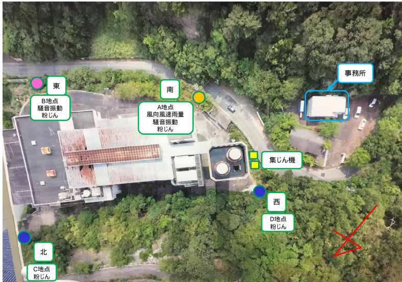
連続粉じんモニタリング設置状況
