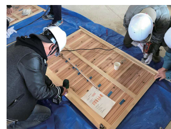
電動工具で木板を固定【外部倉庫WS】
