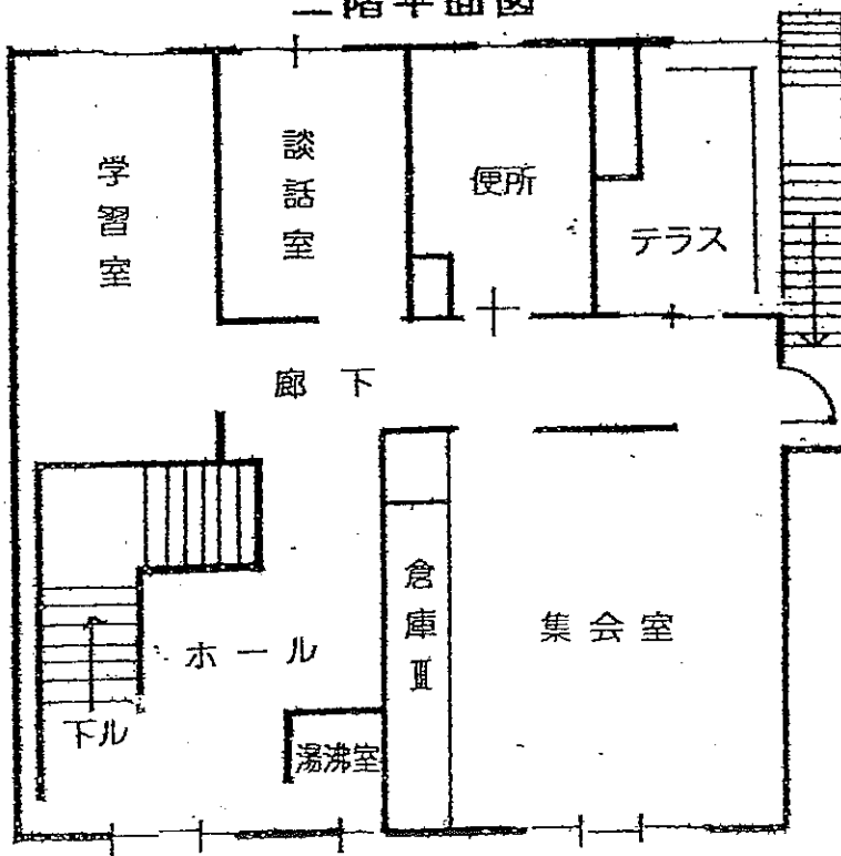
二階平面図
